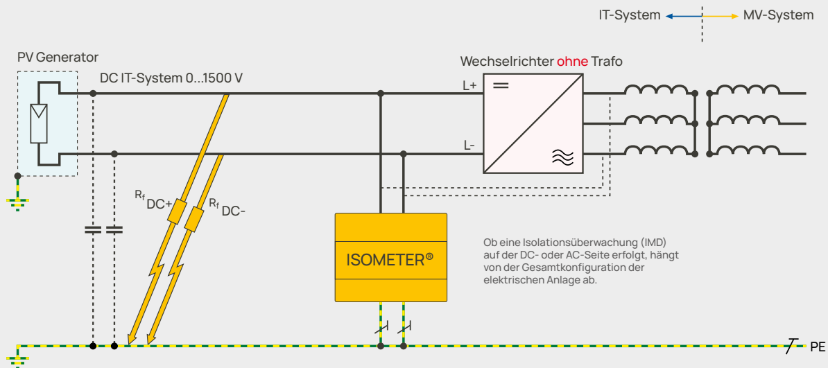
Bild 5: Wechselrichter ohne Transformator
