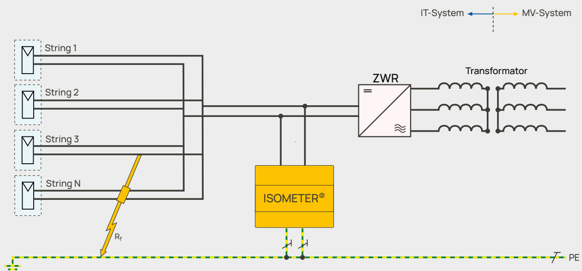
Bild 8: Zentralwechselrichter (ZWR)
