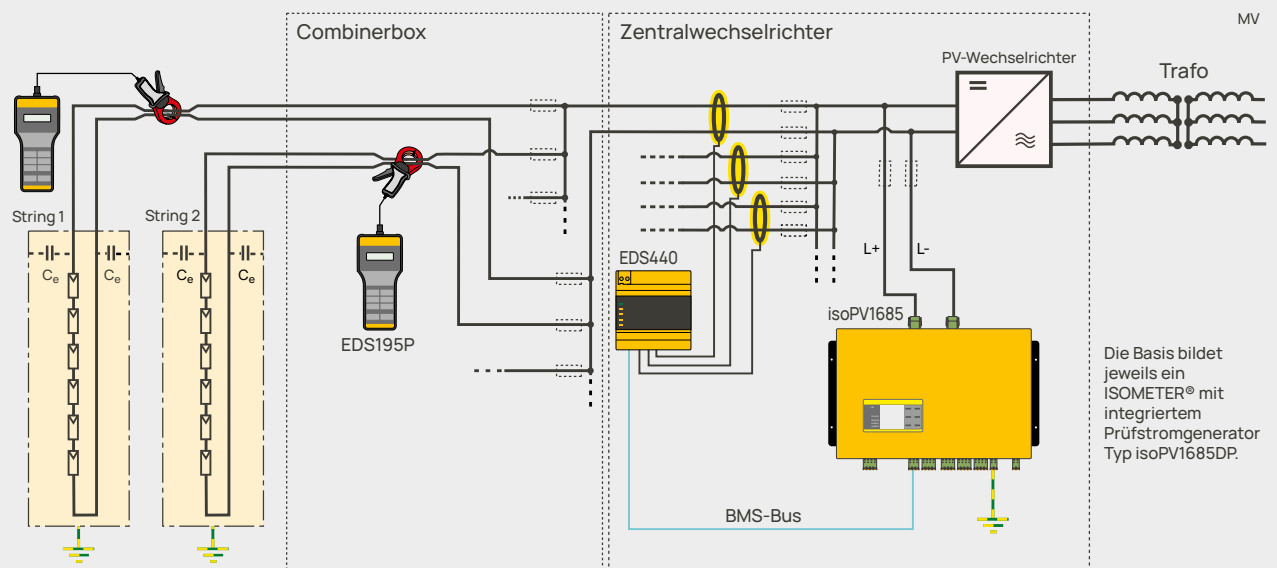
Bild 9: Isolationsfehlersuche mittels fest verbauten Stromwandlern und/oder mobilen Messzangen.
