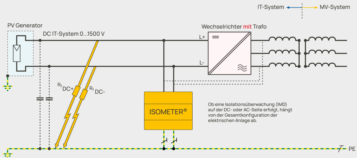
Bild 6: Wechselrichter mit Transformator
