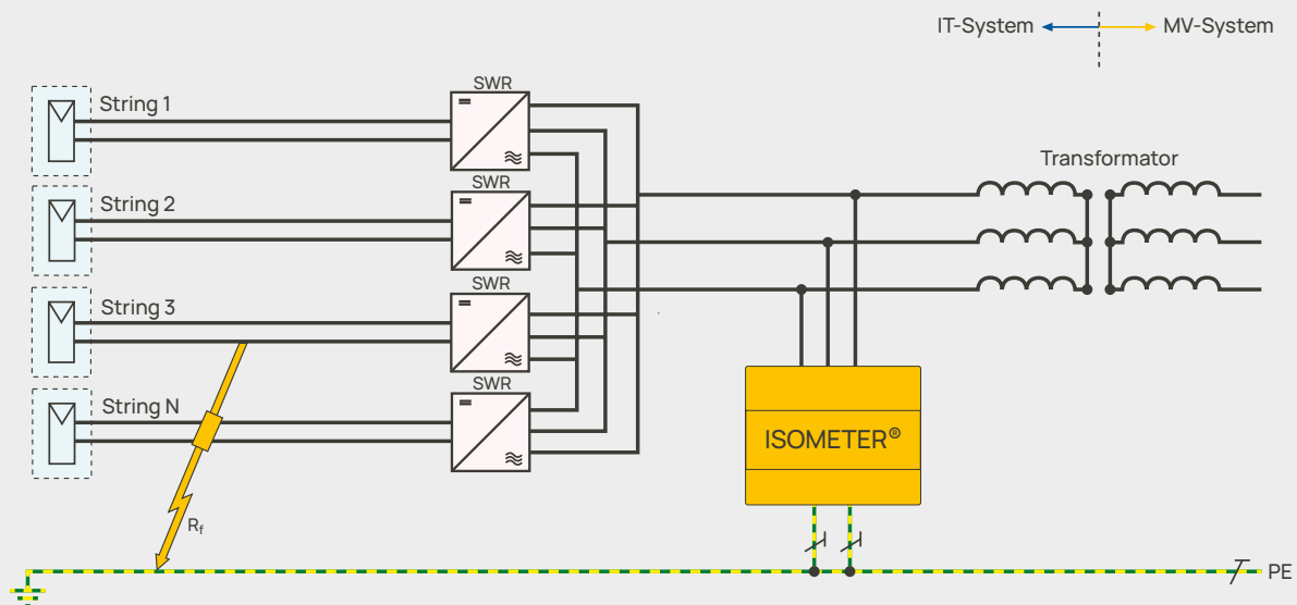
Bild 7: Dezentrale Stringwechselrichter (SWR)
