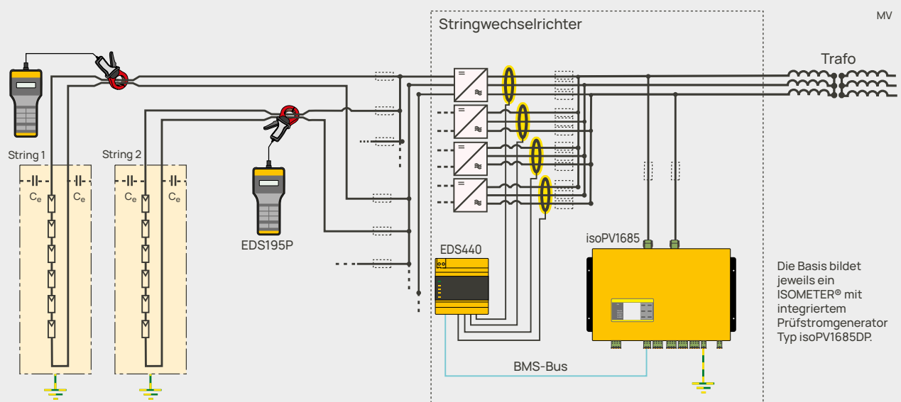
Bild 10: Isolationsfehlersuche mittels fest verbauten Stromwandlern und/oder mobilen Messzangen.
